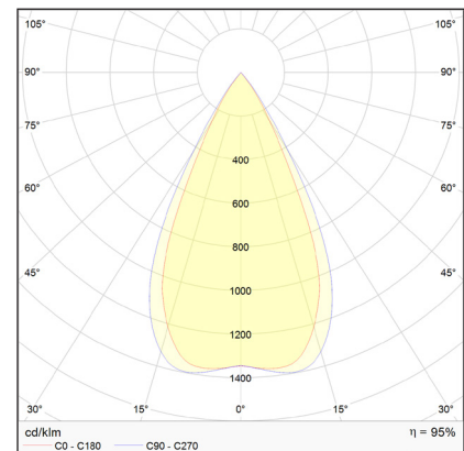
Lichtverteilungskurve CAESAR EL1-D 80° direkt
